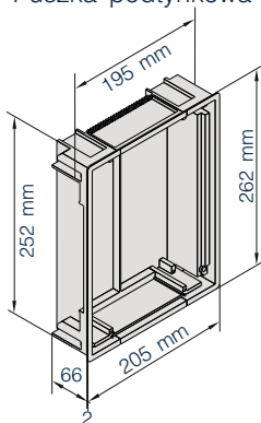
Puszka podtynkowa
