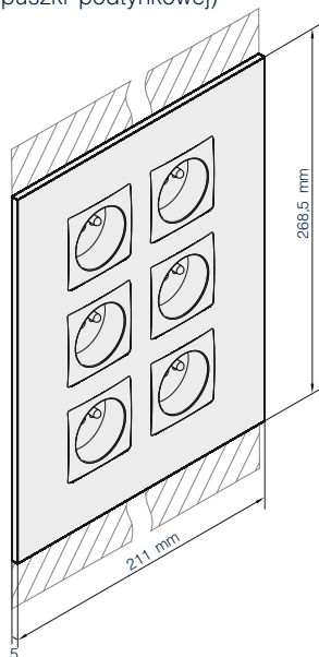
Puszka podtynkowa
