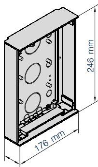
Puszka natynkowa
