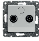
Gniazdo antenowe RTV / Antenna RTv socket pass through przelotowe Tv: 13dB, R: 13dB
